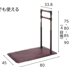
重量 約17.8kg 片手すり BZK-01(N)
