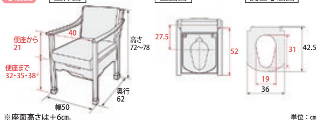
寸法図
